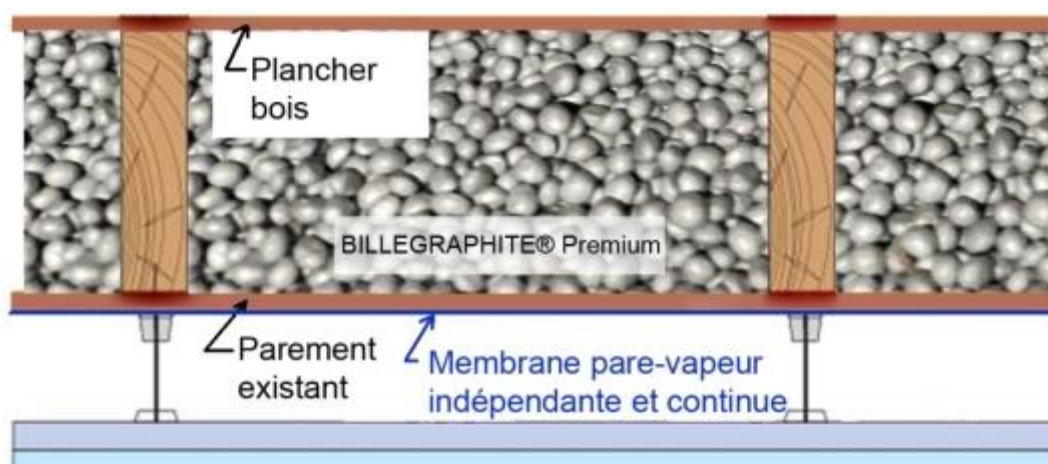
Figure 9 : Pose d'un plenum techniques après la pose du par vapeur après insufflation sur le support à base de plaques de plâtre cartonnées, panneaux de particules de bois ou lambris bois
