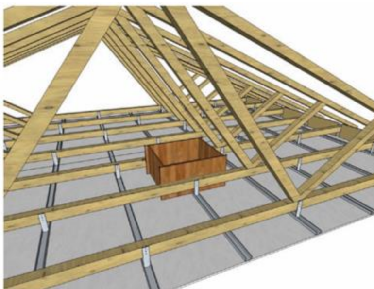
Figure 5 – Traitement des trappes d'accès
